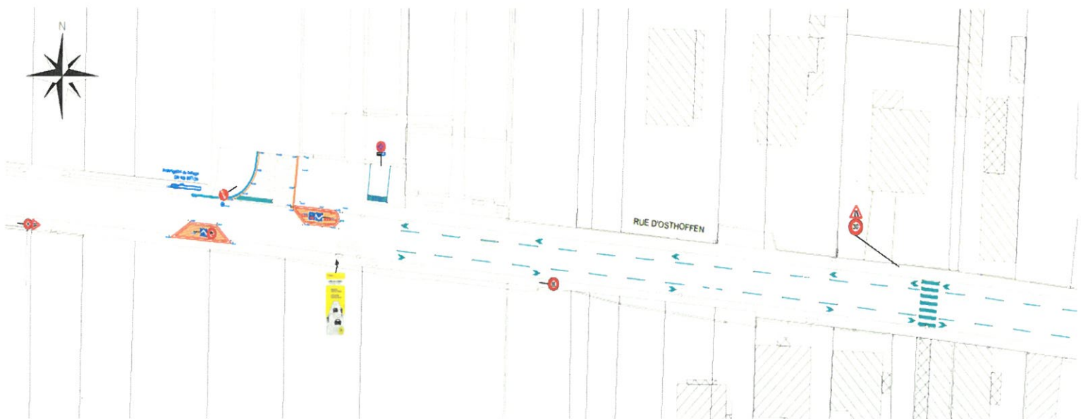
Rue d'Osthoffen : Aménagement de chaussée à voie centrale banalisée
